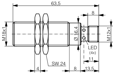
DW-AS-60#-M18-002
